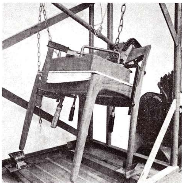
Stole prøves i en speciel prøvemaskine. En god stol skal kunne tåle 50.000 vipninger med 70 kg på sædet.
