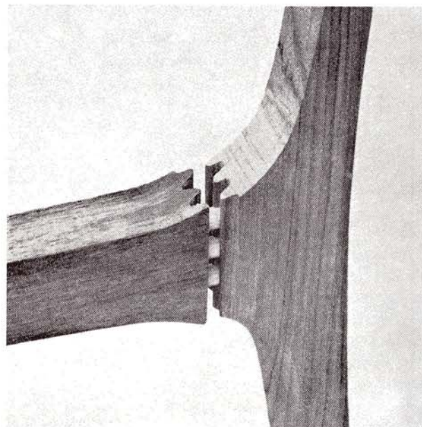
I forbindelse med stoleafprøvningerne foretages i samarbejde med producenterne forbedringer af konstruktionerne, som tilfældet har været med den her viste samling.
